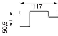
Luftleiste mit den Längen 250 mm, 500 mm, 1.000 mm
