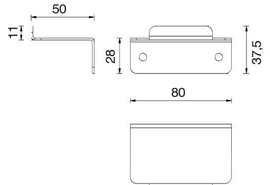
Distanzstück
