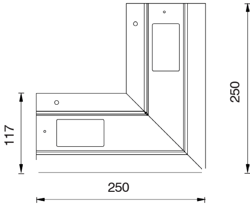
Ecke für Boden oder Wand
