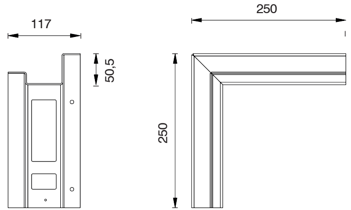
Ecke für Wand oder Decke
