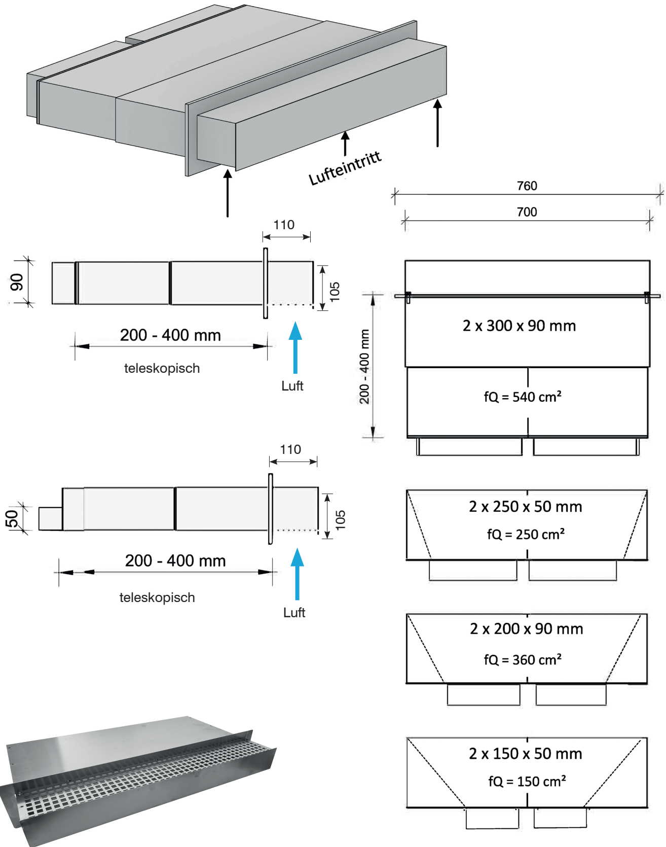
Ansicht von unten
