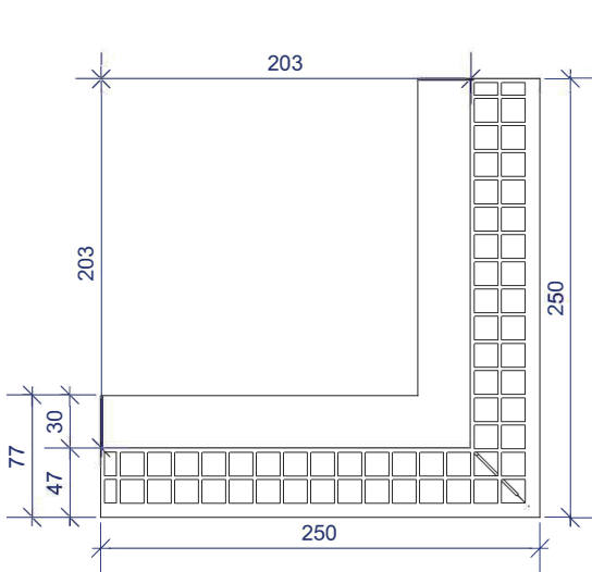
Draufsicht Außenecke
