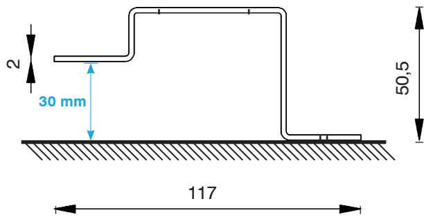
Luftleiste mit den Längen 250 mm, 500 mm, 1.000 mm
