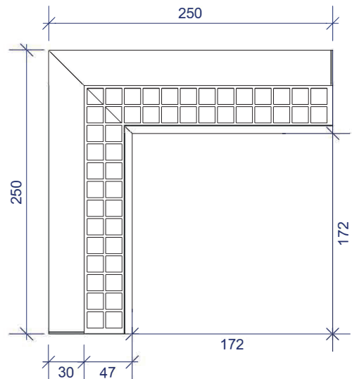
Draufsicht Innenecke
