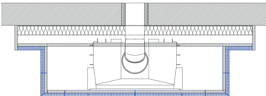
Einbaubeispiel
