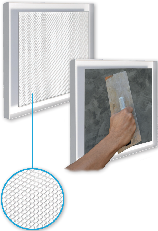
UnderCover „Licht“ mit Putzfront
